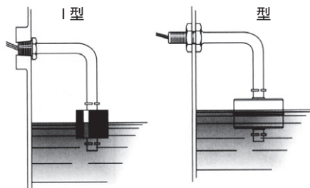
典型安装
